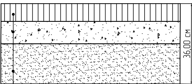
Конструкция демонтажа тротуара из ц/б плитки
