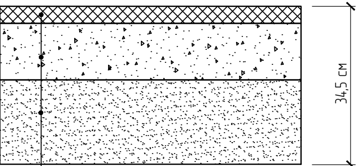
Конструкция демонтажа резинового покрытия
