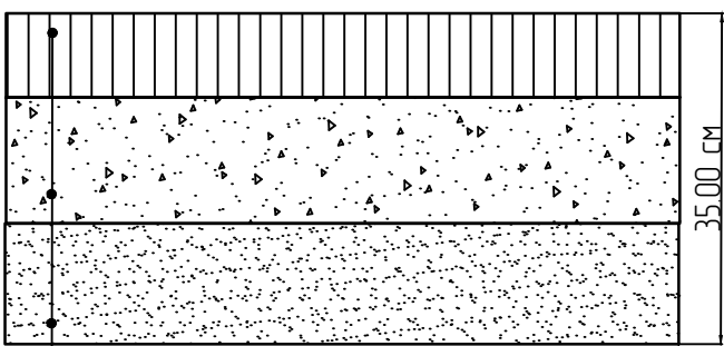
Конструкция демонтажа тротуара из а/б покрытия
